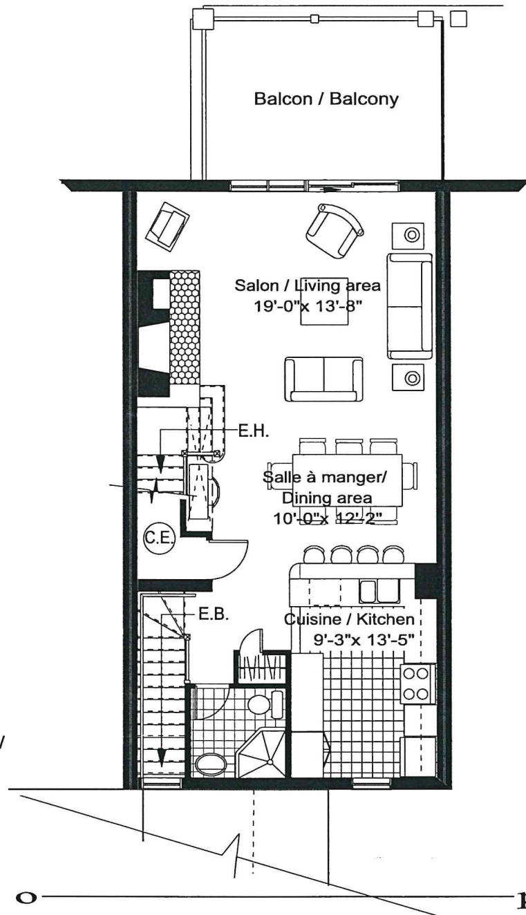
Plan partiel du premier niveau / Partial plan of first level Surface / Area: 61
