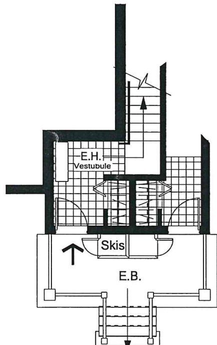
Plan partiel du premier niveau / Partial plan of first level Surface / Area: 61
